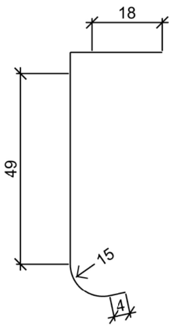
Seitensicht
